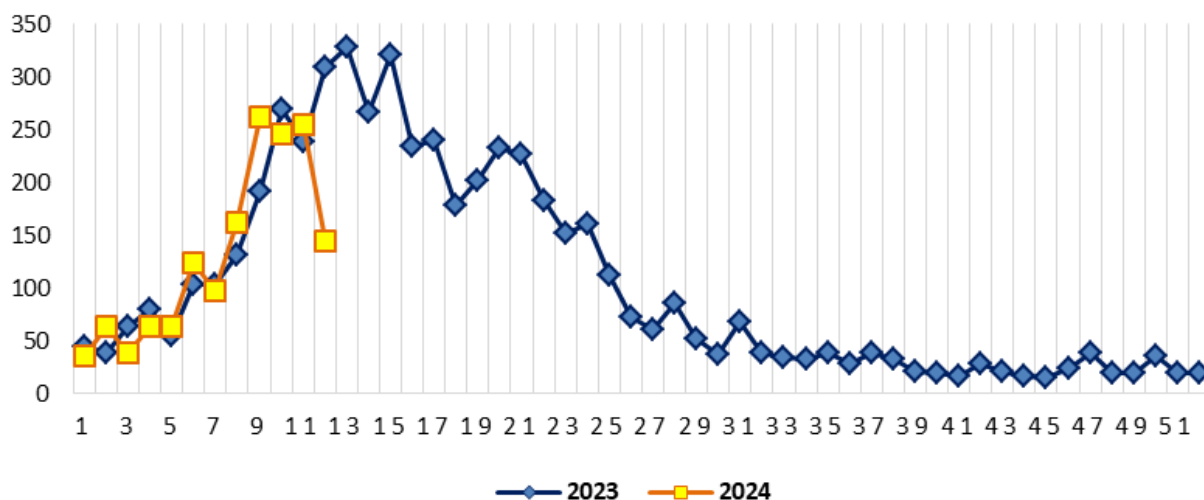
Gráfico 2: Variação dos casos de dengue segundo semana epidemiológica no ano de 2024 em Teresina
